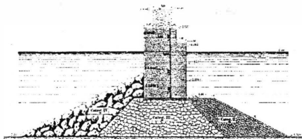
PROFIL №1
